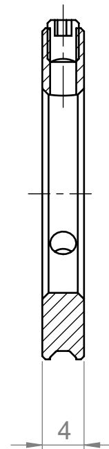
A-A SCALE 2 : 1
